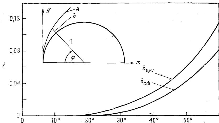
Рис. 8.13. Длина стебля Маха для вторичной ударной волны. A — вторичная ударная волна. По оси абсцисс отложены значения \varphi .
