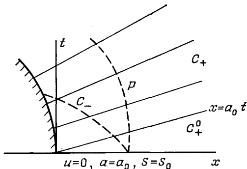
Рис. 6.1. Волна разрежения, возникающая при вытягивании поршня.
