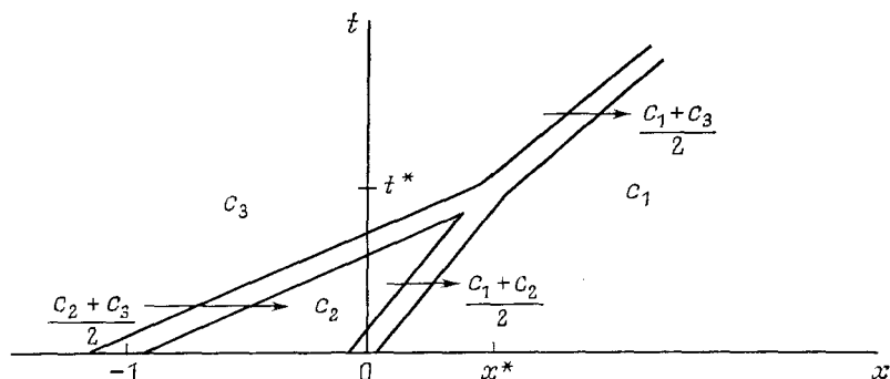
Рис. 4.3. Сливающиеся ударные волны.
