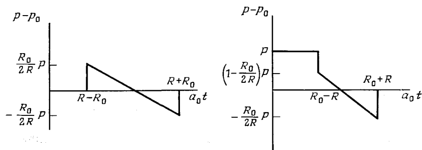
Рис. 7.1. Картина давления в задаче о взрыве шара.
