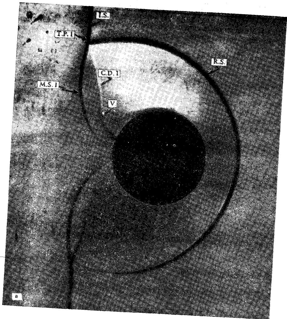
Рис. 8.15а. Теневая фотография дифракции ударной волны на цилиндре диаметром 0,5 дюйма (1,27 см) при M_0 = 2,82 . Видна начальная стадия отрыва пограничного слоя. (По Брисону и Гроссу [1]).
