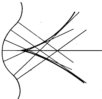
Рис. 7.9. Образование каустики.
