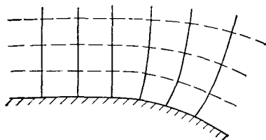
Рис. 8.2. Положения ударной волны (сплошные кривые) и лучей (штриховые кривые) при дифракции ударной волны на закругленном угле.
