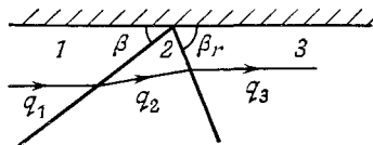
Рис. 6.13. Регулярное отражение ударной волны.
