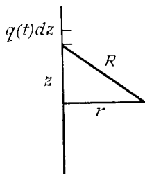
Рис. 7.2. Детали построения для линейного источника.
