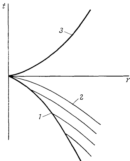
Рис. 6.8. (r, t) -диаграмма для сходящейся ударной волны.
