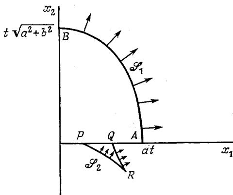
Рис. 7.14. Волновые фронты в магнитной газовой динамике.
