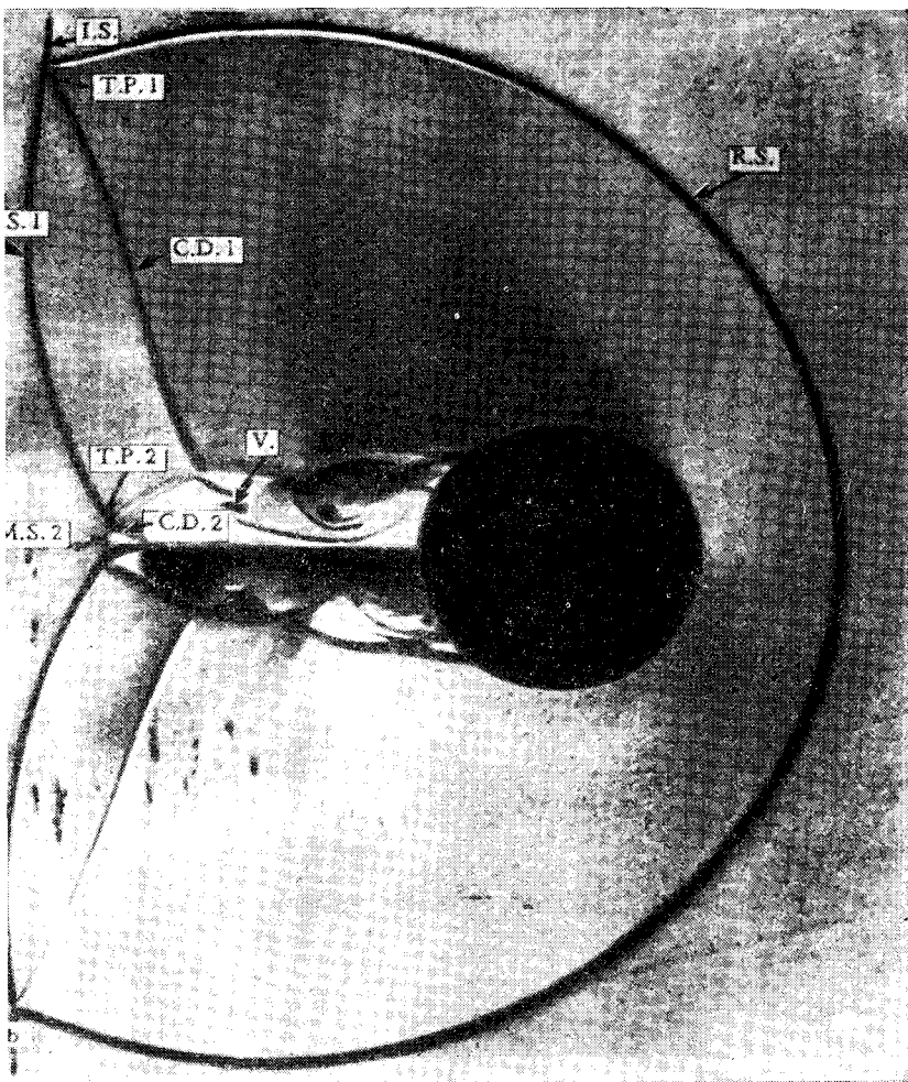
8.15b. Теневая фотография дифракции ударной волны на цилиндре диаметром 0,5 дюйма при M_0 = 2,81 . (По Брисону и Гроссу [1]). Обозначения те же, что на рис. 8.15а.
