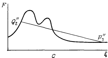
Рис. 2.16. Построение сливающихся разрывов.
