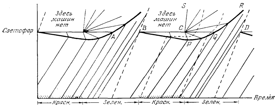
Рис. 3.3. Волновая диаграмма для задачи о светофоре.
