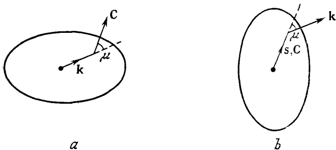
Рис. 12.10. a — дисперсионная поверхность в \mathbf{k} -пространстве, b — фазовая поверхность в \mathbf{x} -пространстве.
