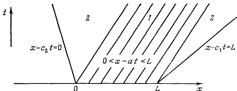
Рис. 10.1. (x, t) -диаграмма для задачи Коши. 1 — основное возмущение, 2 — малые возмущения.
