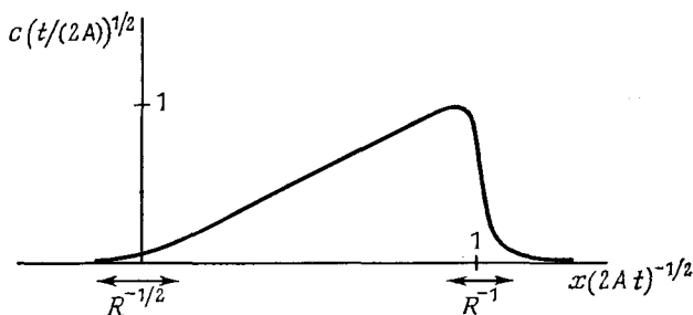
Рис. 4.1. Решение уравнения Бюргера в виде треугольной волны.
