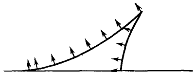
Рис. 12.5. Линия гребня в задаче о корабельных волнах.
