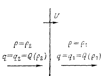
Рис. 2.5. Параметры течения для движущегося разрыва.
