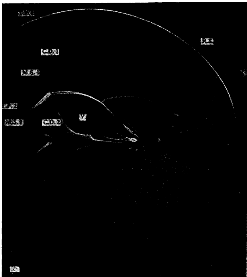
Рис. 8.15с. Теневая фотография дифракции ударной волны на цилиндре диаметром 0,5 дюйма при M_0 = 2,84 . (По Брисону и Гроссу [1].) Обозначения те же, что на рис. 8.15а.
