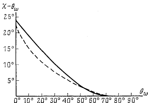
Рис. 8.11. Зависимость угла \chi - \theta_w от угла клина \theta_w для отражения Маха. Сплошная кривая соответствует данной теории, штриховая — теории с тремя ударными волнами.
