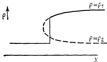
Рис. 3.6. Структура ударной волны с внутренним разрывом.
