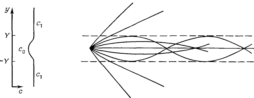
Рис. 7.10. Волновод в океане.
