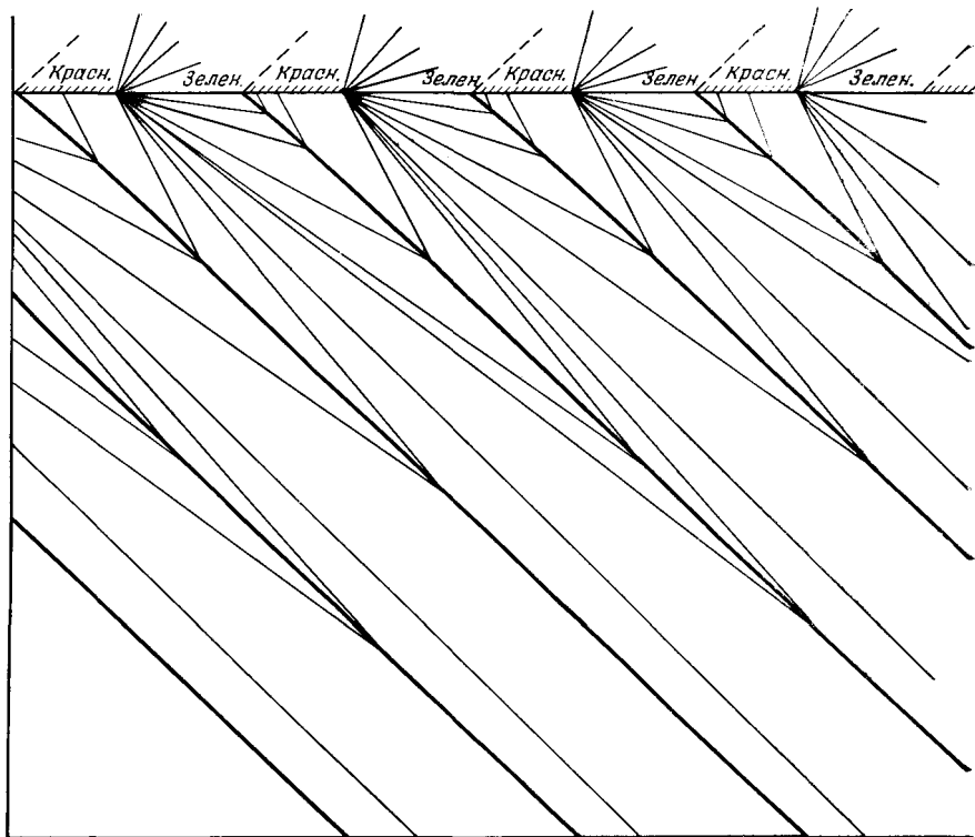
Рис. 3.4. Волновая диаграмма для эле движущегося потока транспорта у перегруженного светофора.
