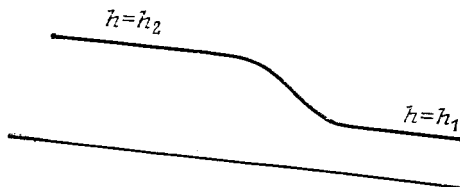
Рис. 3.8. Структура моноклиальной паводковой волны.
