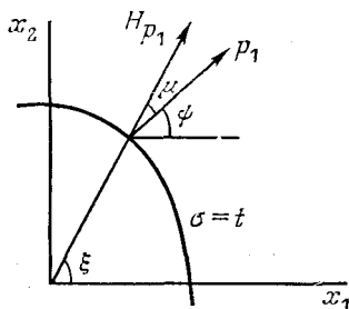
Рис. 7.13. Геометрия волнового фронта, лучей и нормалей в анизотропной среде.
