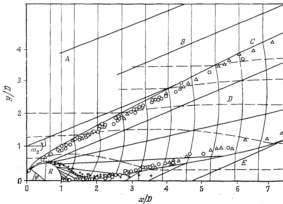
Рис. 8.14. Дифракция на цилиндре при M_0 = 2,81 (по Брисону и Гроссу [11]). A — экспериментально найденные тройные точки, B — характеристики, C — вторичная ударная волна 1, D — лучи, E — вторичная ударная волна 2.
