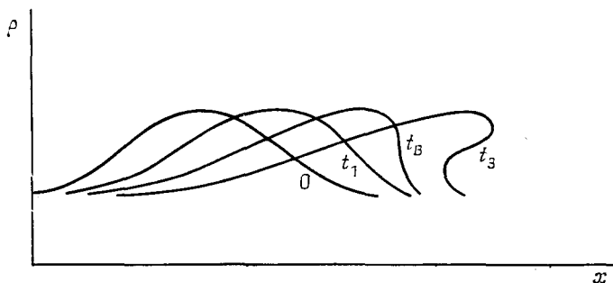
Рис. 2.2. Опрокидывающаяся волна. Построены профили, соответствующие моментам времени 0, t_1, t_B, t_3 (см. рис. 2.1).
