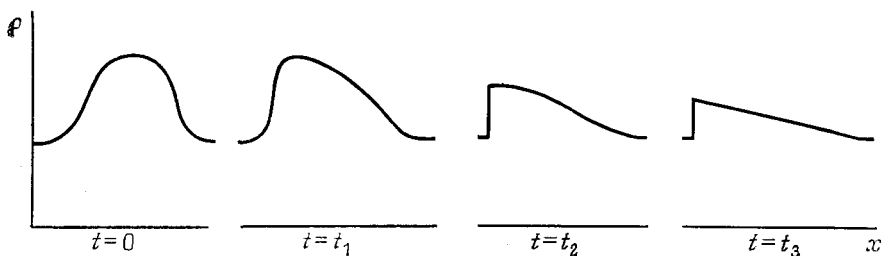
Рис. 3.2. Опрокидывание волны в потоке транспорта.
