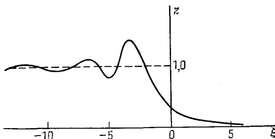
Рис. 13.6. Модель структуры борма. Решение уравнения (13.139) для m = 1/2 .
