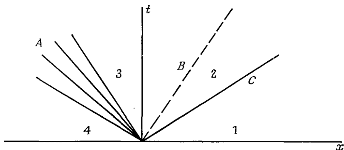
Рис. 6.5. (x, t) -диаграмма для ударной трубы.
